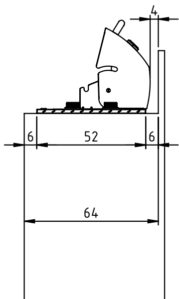
VISTA LATERAL
