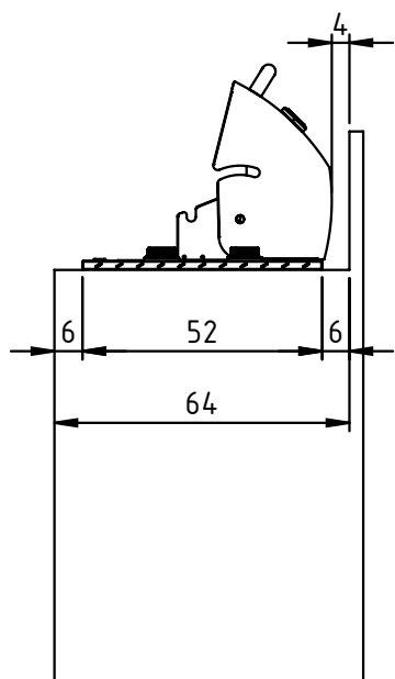
VISTA LATERAL
